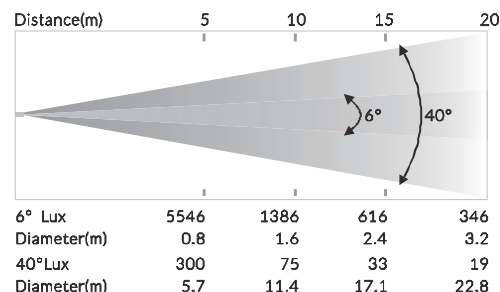
照度図
