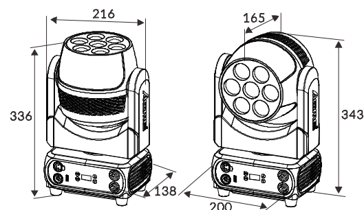
寸法図(mm)
