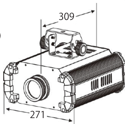
寸法図(mm)
