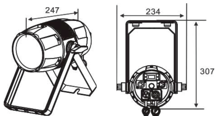
寸法図(mm)
