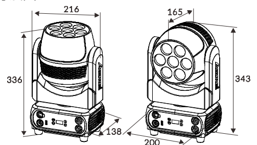
寸法図
