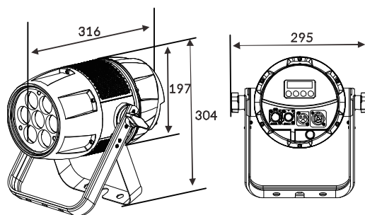
寸法図(mm)
