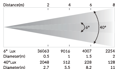
照度図
