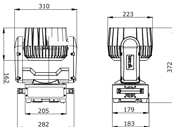
寸法図
