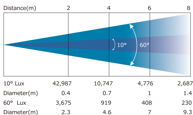
照度図
